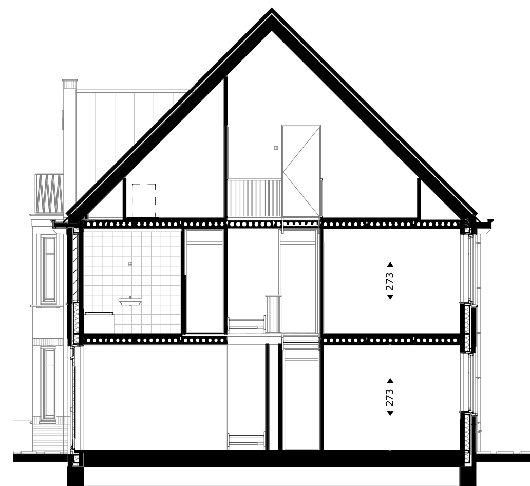
doorsnede A-A
