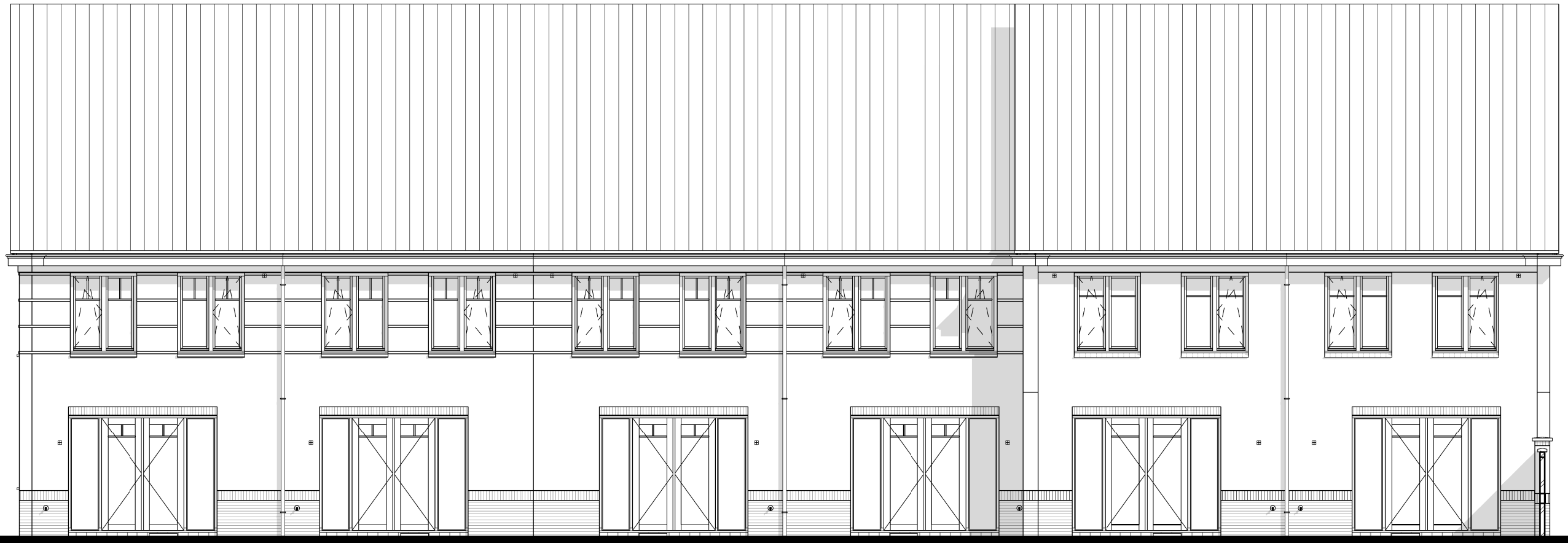
BNR 90 BNR 89 BNR 88 BNR 87 BNR 86 BNR 85 achtergevel
