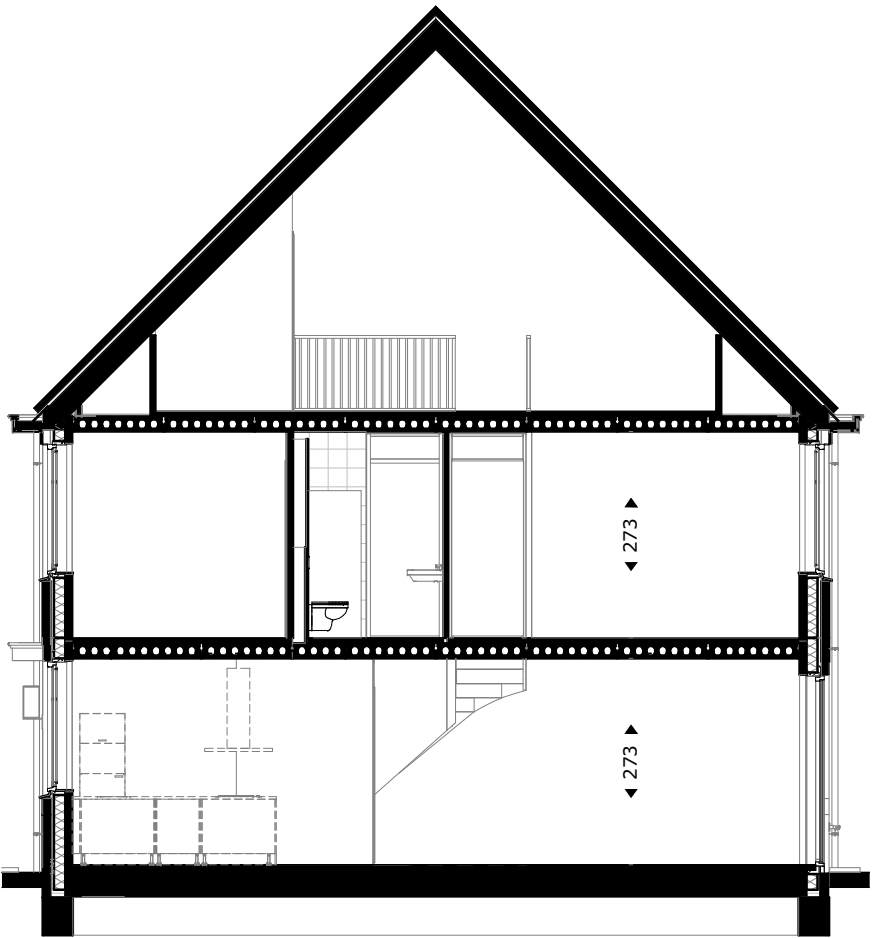
doorsnede A-A
