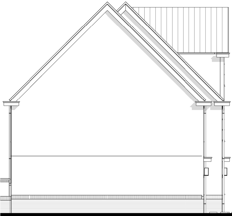
BNR 85 linker zijgevel
