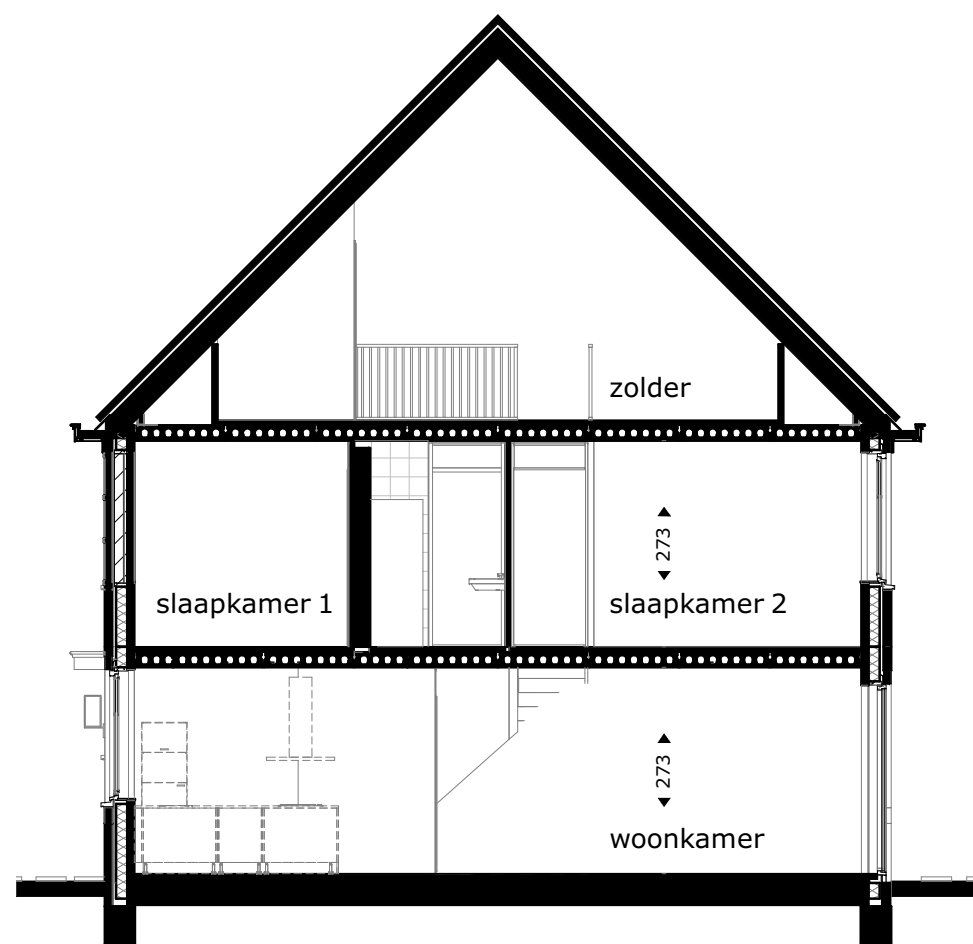
doorsnede A-A
