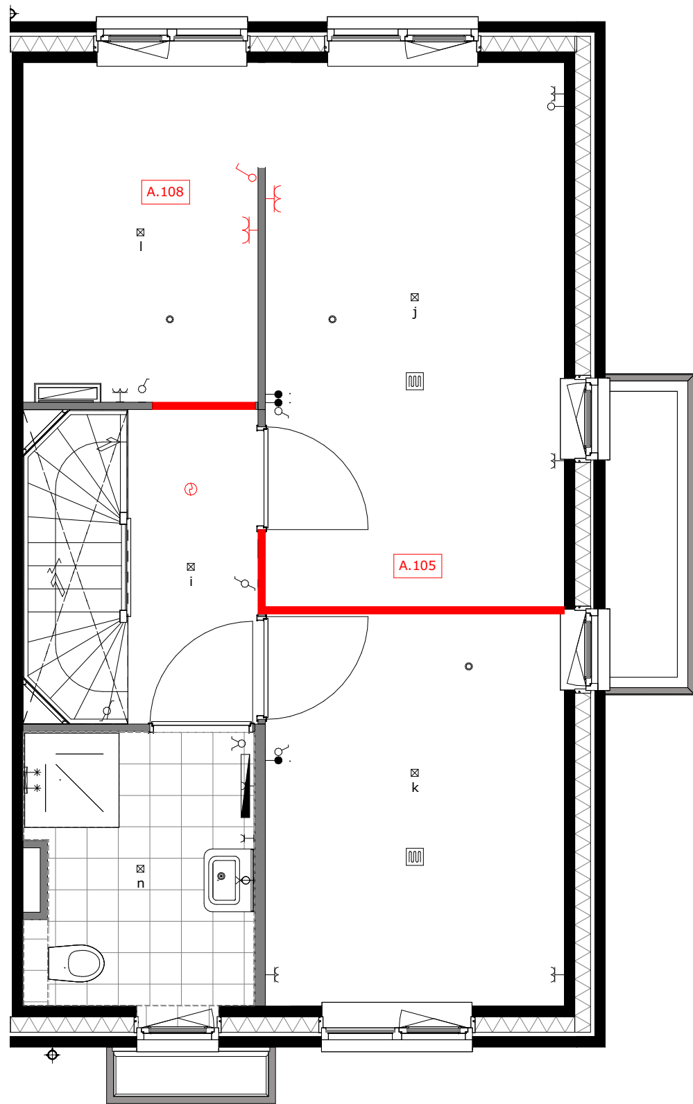
A.105 = verplaatsen wand slaapkamer 1 en 2 A.108 = slaapkamer 1 met inloopkast
