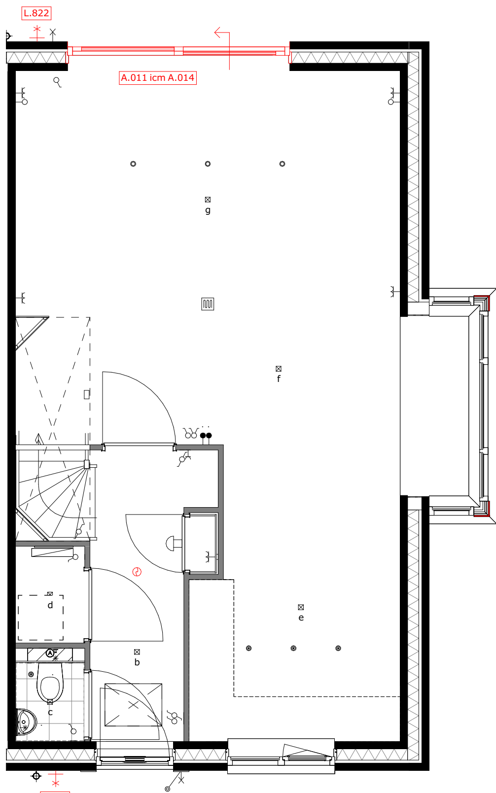
A.014 = wijzigen schuivende deel icm. optie A.011 L.820 = buitenkraan voorgevel L.822 = buitenkraan achtergevel
