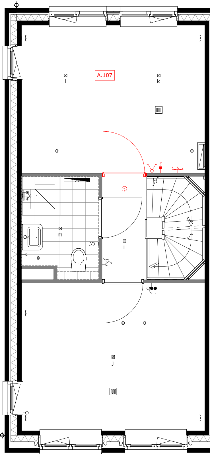
A.107 = samenvoegen slaapkamer 2 en 3
