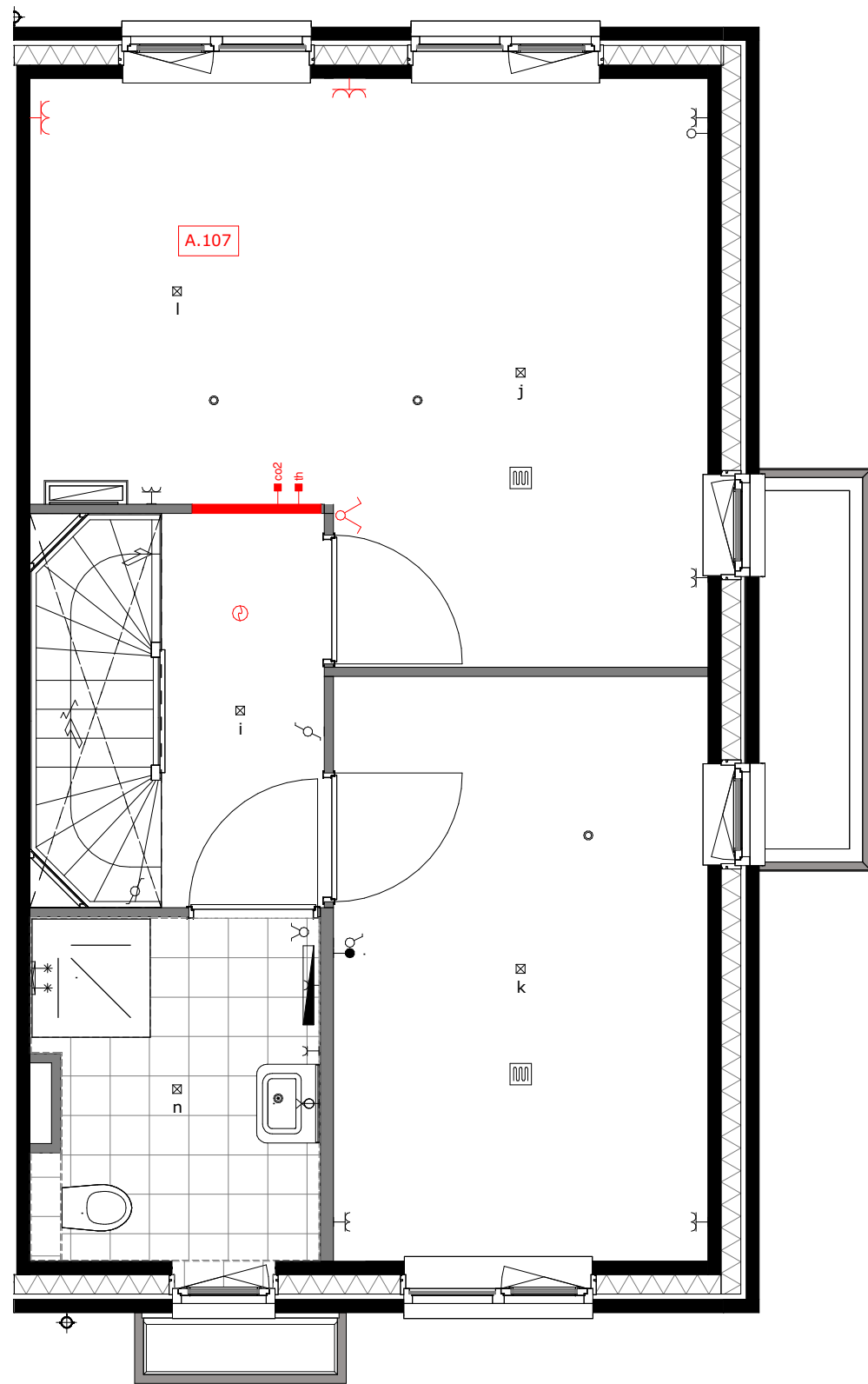
A.107 = slaapkamer 1 en 3 samenvoegen
