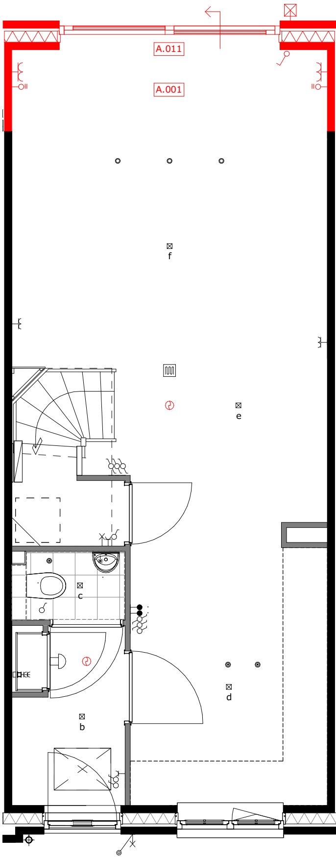
A.001 = uitbouw 1.2m A.011 = schuifpui
