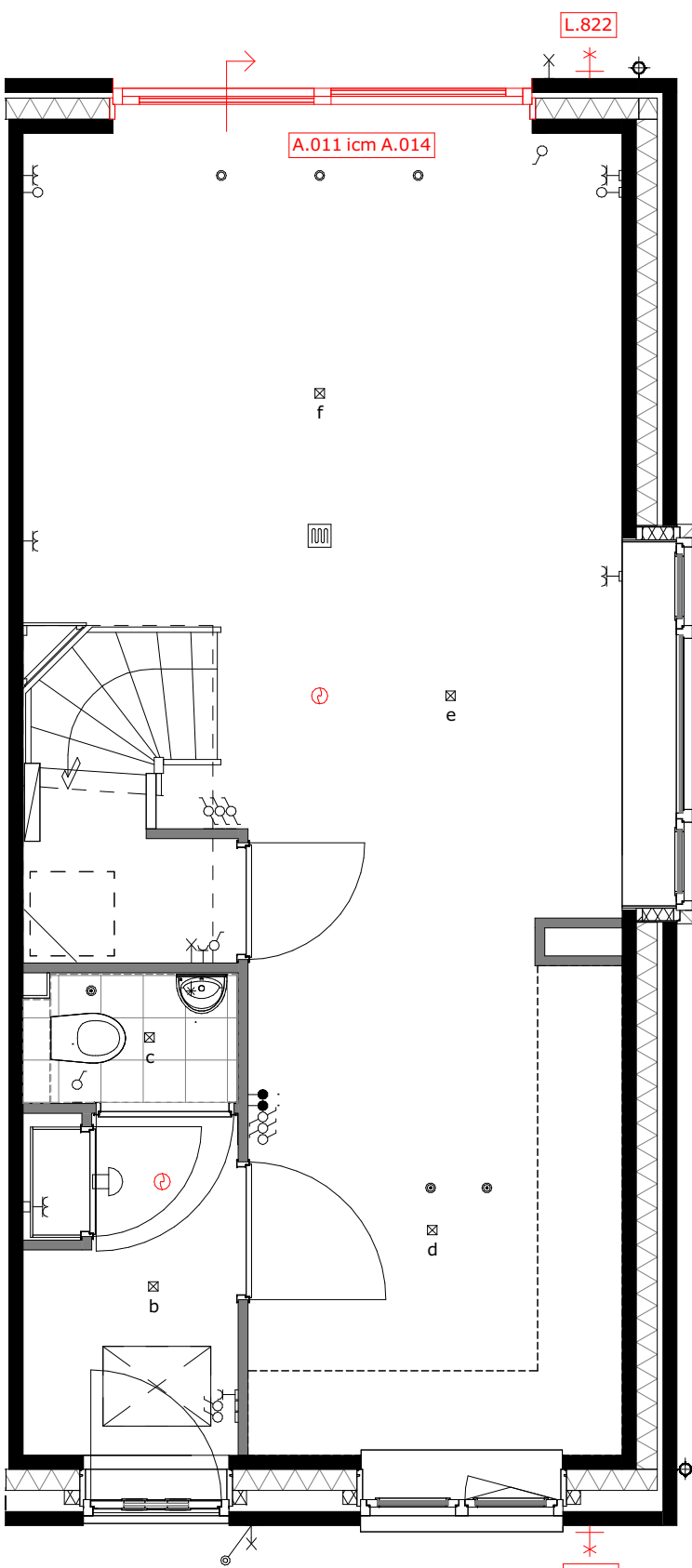
A.014 = wijzigen schuivende deel icm. optie A.011 L.820 = buitenkraan voorgevel L.822 = buitenkraan achtergevel
