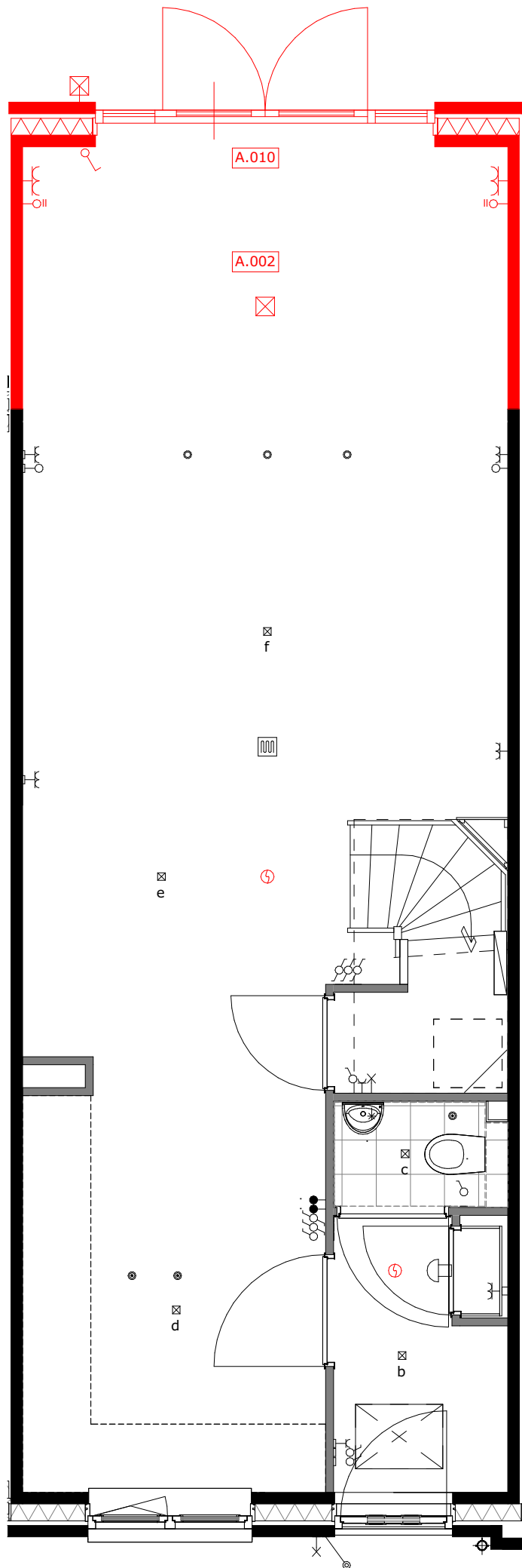
A.002 = uitbouw 2.4m A.010 = openslaande deuren
