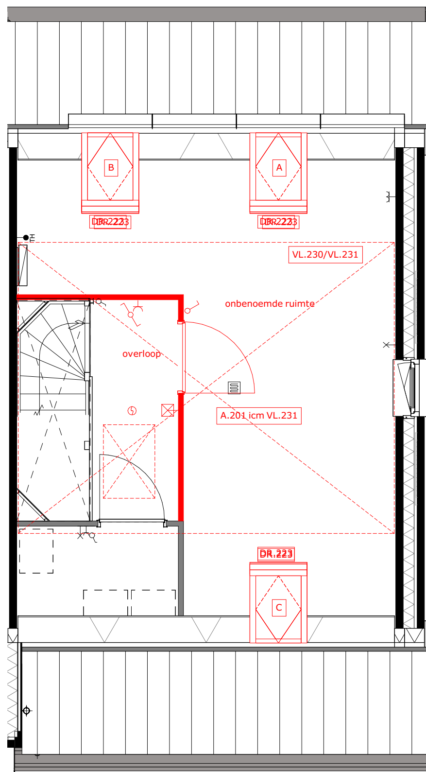
A.201 = zolderindeling (alleen in combinatie met VL.231) DR.223 = houten tuimeldakraam VL.230 = vliering (onafgewerkt) VL.231 = vliering afgewerkt
