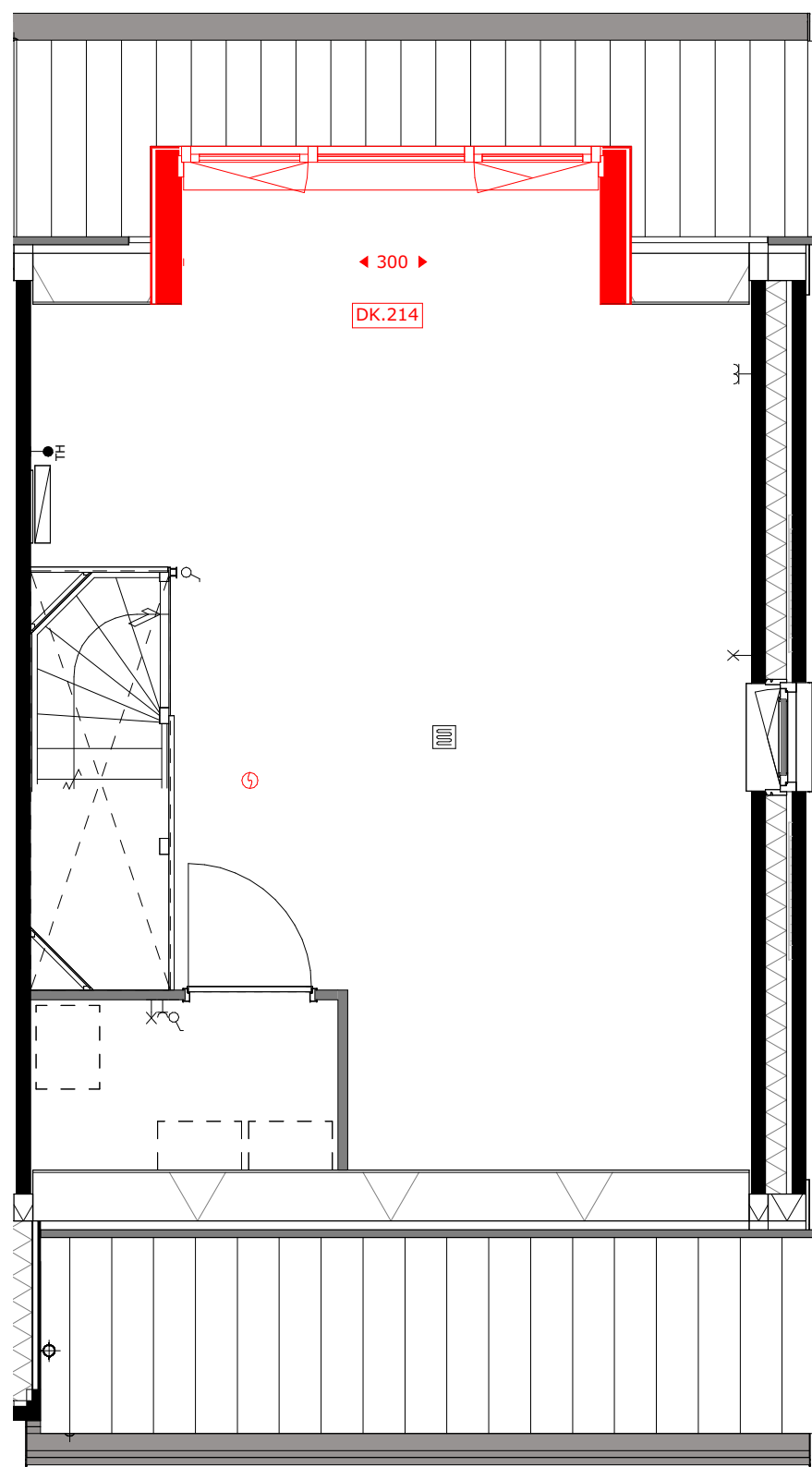
DK.214 = dakkapel achtergevel (breedte c.a. 3m)
