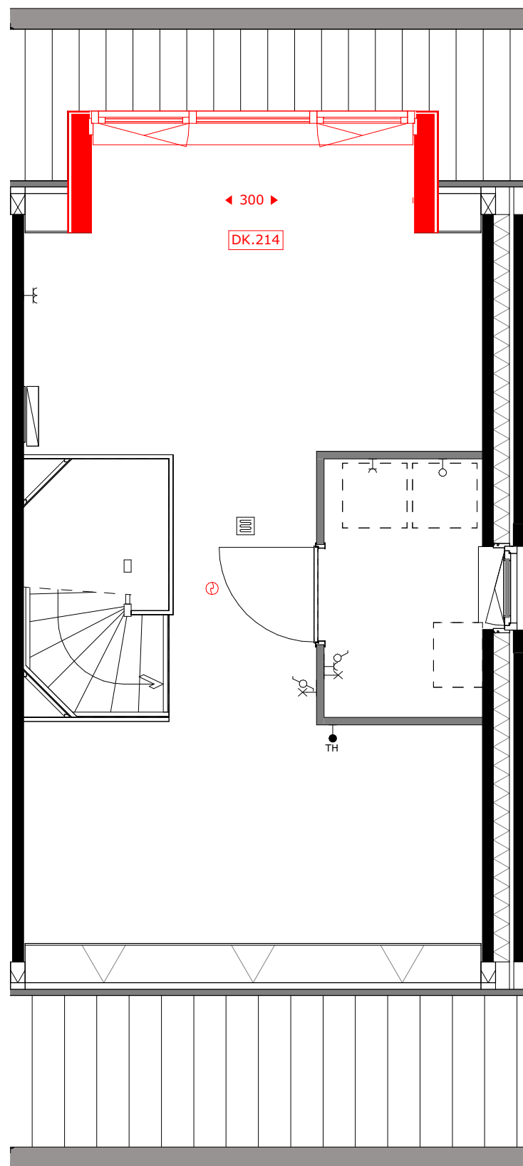
DK.214 = dakkapel achtergevel (breedte c.a. 3m)
