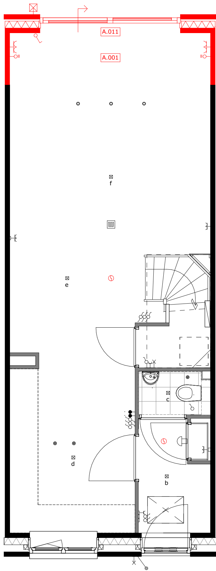
A.001 = uitbouw 1.2m A.011 = schuifpui
