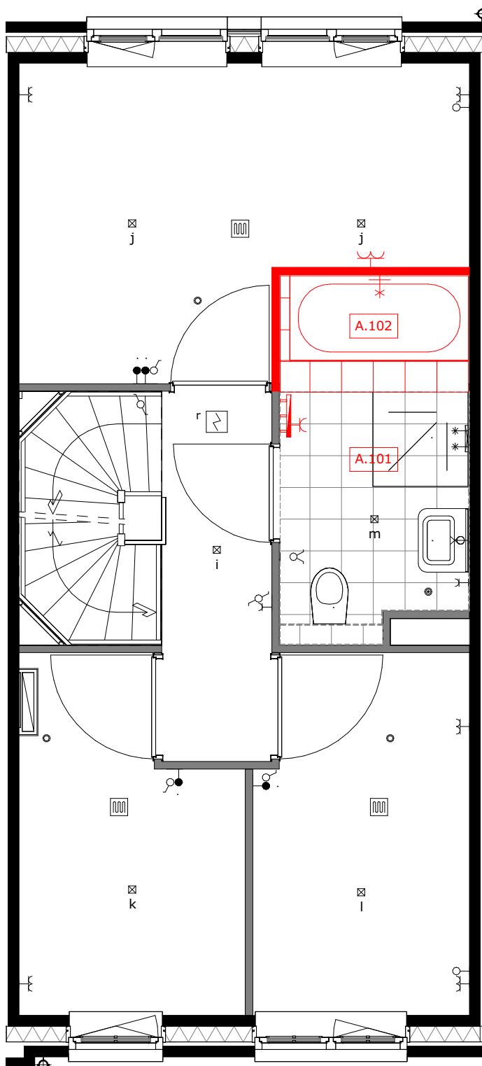
A.101 = vergroten badkamer ca. 110cm A.102 = ligbad met plateau, alleen mogelijk icm optie A.101
