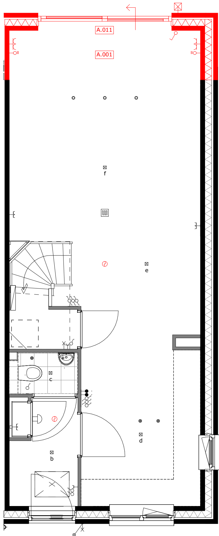
A.001 = uitbouw 1.2m A.011 = schuifpui
