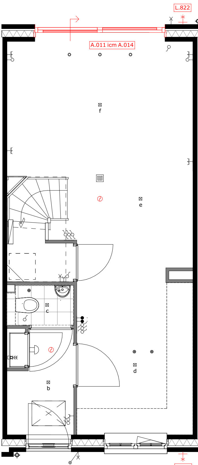
A.014 = wijzigen schuivende deel icm. optie A.011 L.820 = buitenkraan voorgevel L.822 = buitenkraan achtergevel
