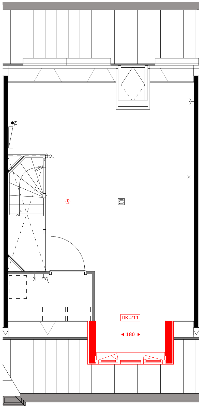
DK.211 = dakkapel voorgevel (breedte c.a. 1.8m)
