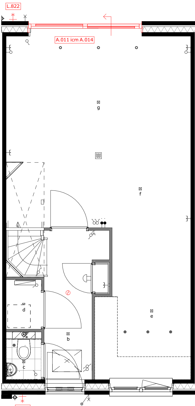
A.014 = wijzigen schuivende deel icm. optie A.011 L.820 = buitenkraan voorgevel L.822 = buitenkraan achtergevel
