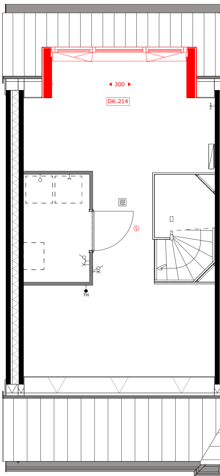
DK.214 = dakkapel achtergevel (breedte c.a. 3m)
