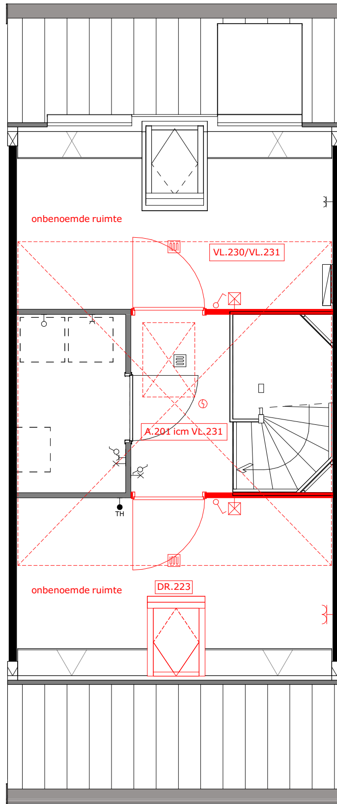
A.201 = zolderindeling (alleen in combinatie met VL.231) DR.223 = dakvenster VL.230 = vliering (onafgewerkt) VL.231 = vliering afgewerkt
