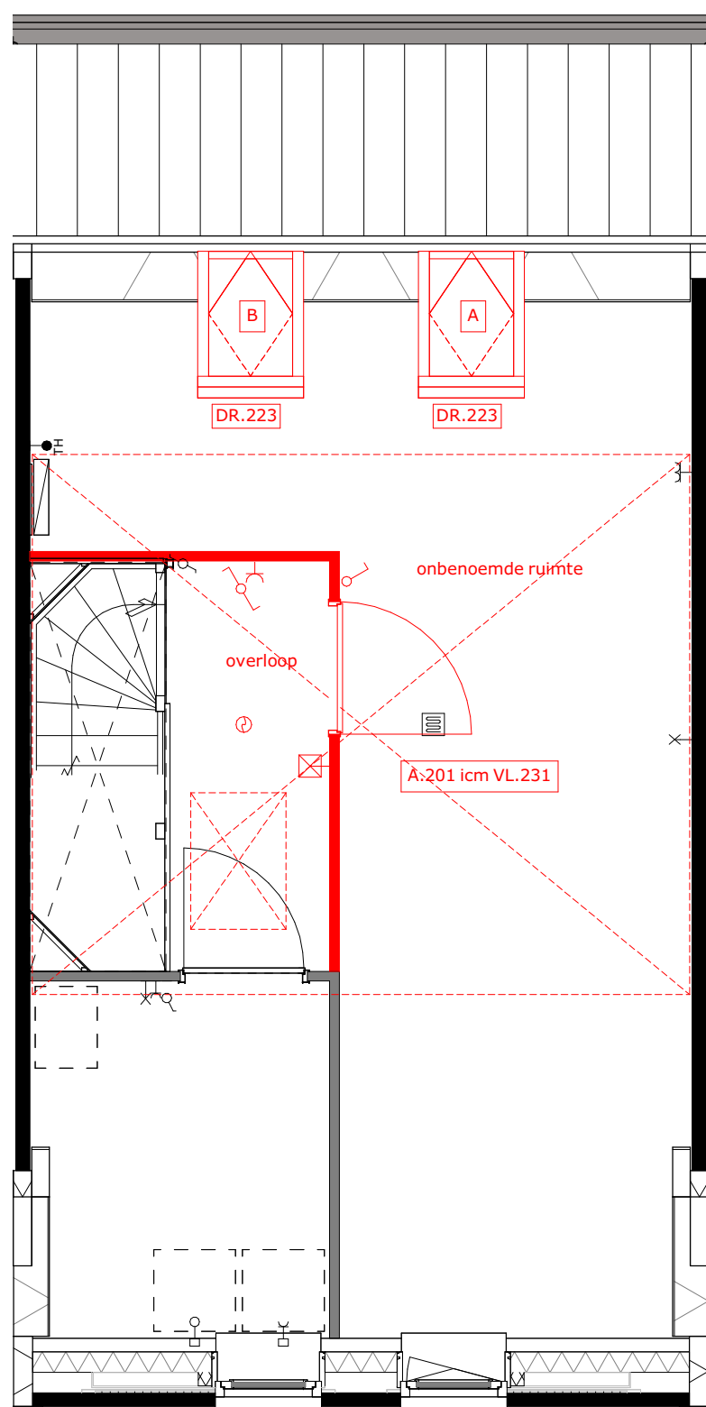
A.201 = zolderindeling (alleen in combinatie met VL.231) DR.223 = houten tuimeldakraam VL.230 = vlIERING (onafgewerkt) VL.231 = vlIERING afgewerkt
