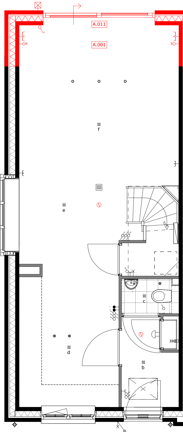
A.001 = uitbouw 1.2m A.011 = schuifpui
