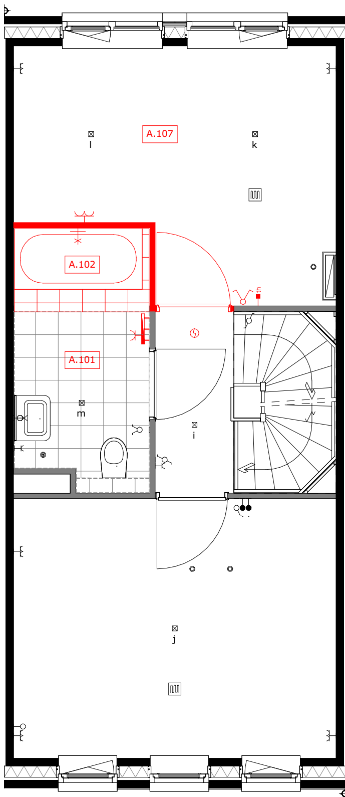
A.101 = vergroten badkamer ca. 110cm, alleen mogelijk icm optie A.107 A.102 = ligbad met plateau, alleen mogelijk icm optie A.101 A.107 = samenvoegen slaapkamer 2 en 3
