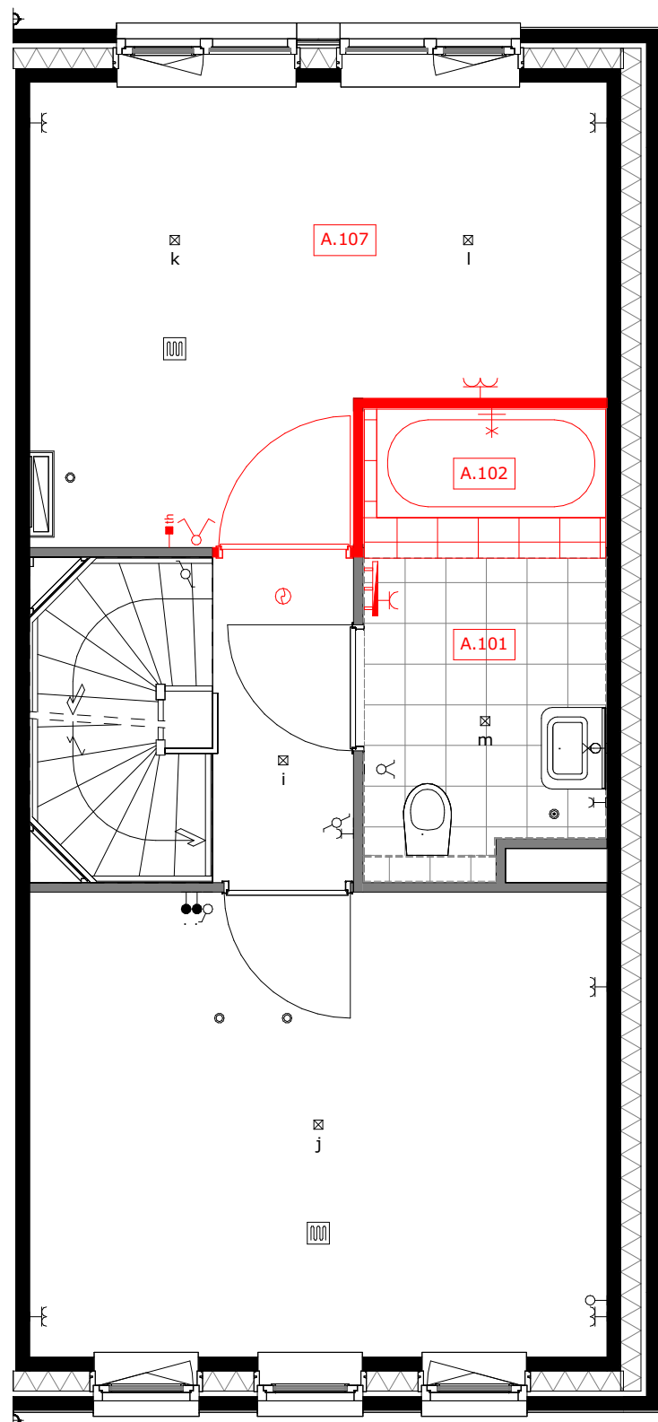
A.101 = vergroten badkamer ca. 110cm, alleen mogelijk icm optie A.107 A.102 = ligbad met plateau, alleen mogelijk icm optie A.101 A.107 = samenvoegen slaapkamer 2 en 3
