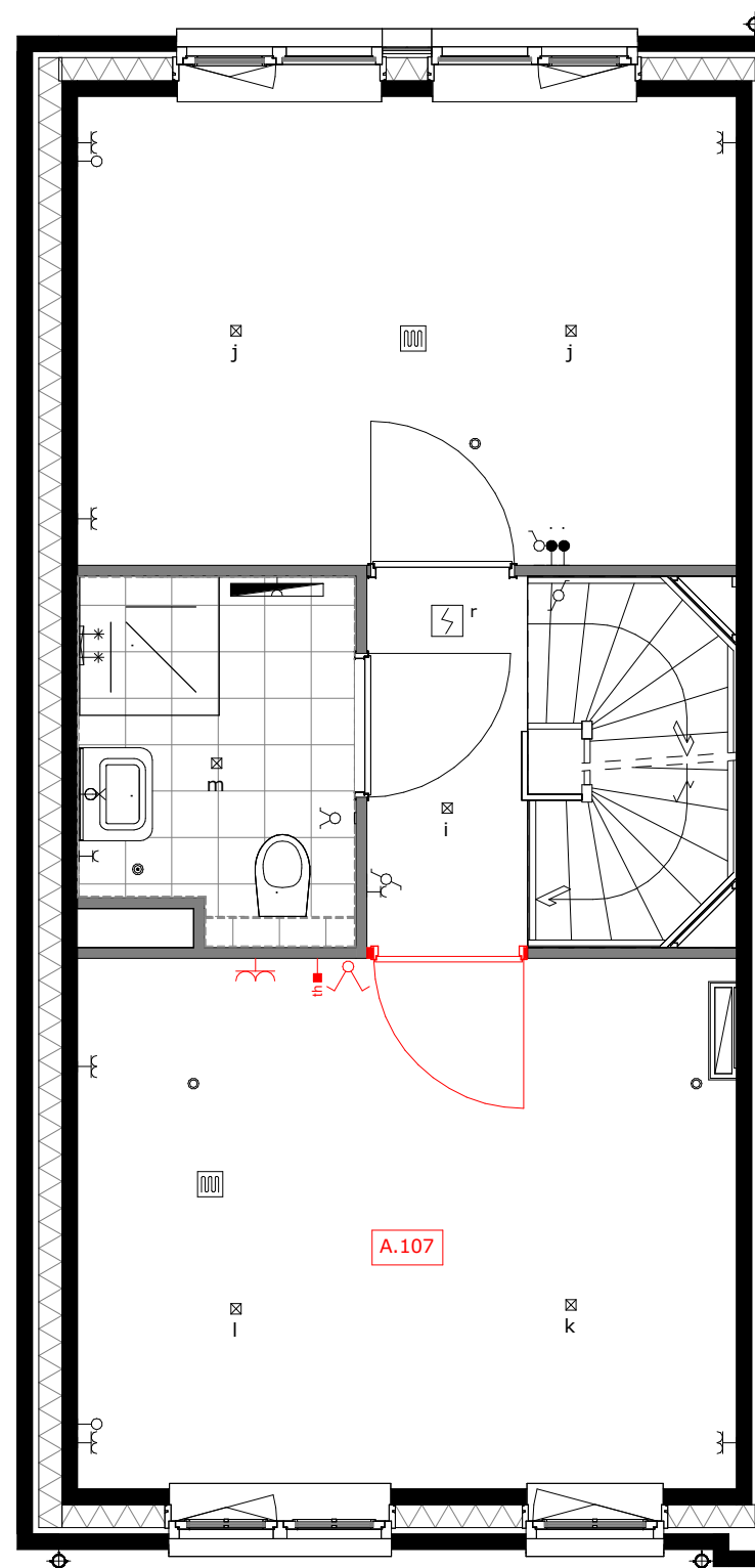
A.107 = samenvoegen slaapkamer 2 en 3
