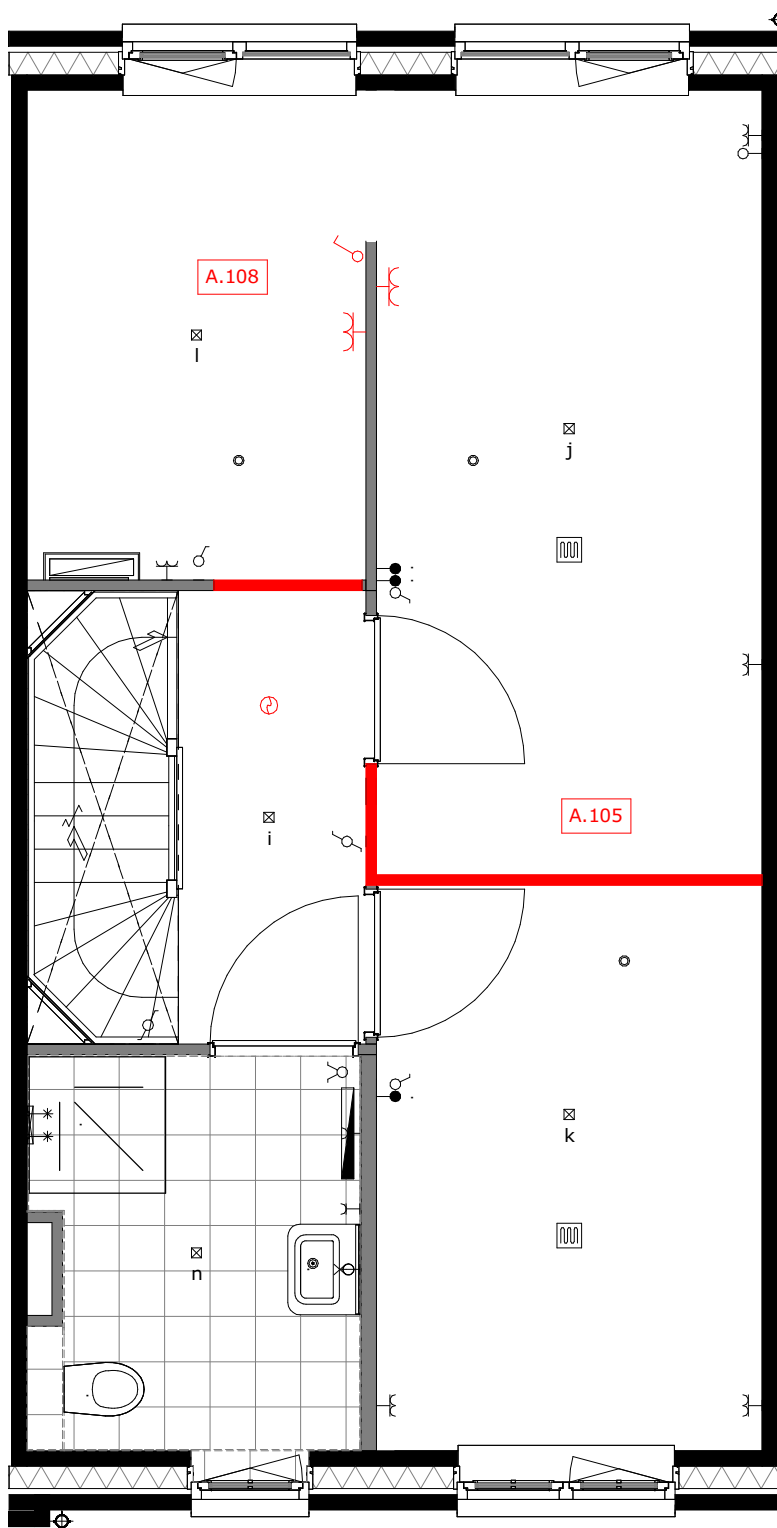
A.105 = verplaatsen wand slaapkamer 1 en 2 A.108 = slaapkamer 1 met inloopkast
