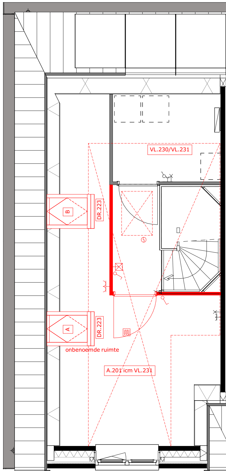
A.201 = zolderindeling (alleen in combinatie met VL.231) DR.223 = dakvenster VL.230 = vliering (onafgewerkt) VL.231 = vliering afgewerkt
