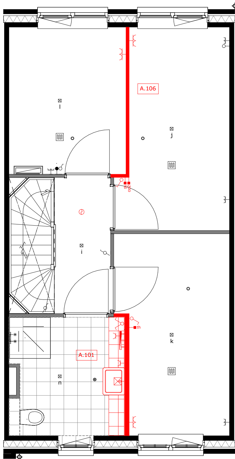
A.101 = vergroten badkamer ca. 35cm A.106 = verplaatsen wand slaapkamer 1 en 3
