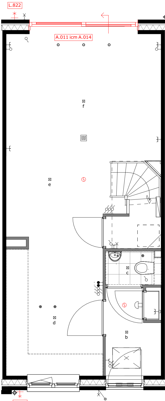
A.014 = wijzigen schuivende deel icm. optie A.011 L.820 = buitenkraan voorgevel L.822 = buitenkraan achtergevel
