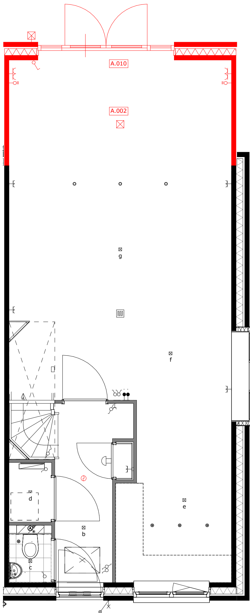
A.002 = uitbouw 2.4m A.010 = openslaande deuren
