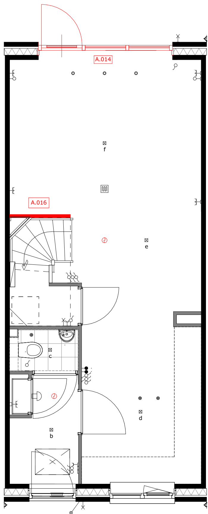
A.014 = wijzigen loopdeur A.016 = wand bij de trap
