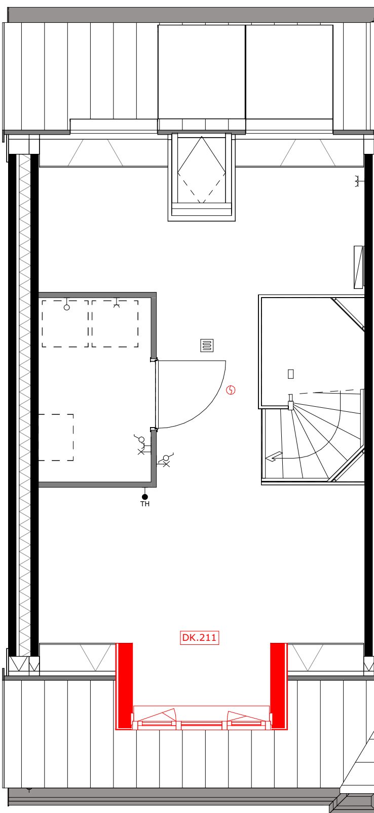
DK.211 = dakkapel voorgevel (breedte c.a. 1.8m)
