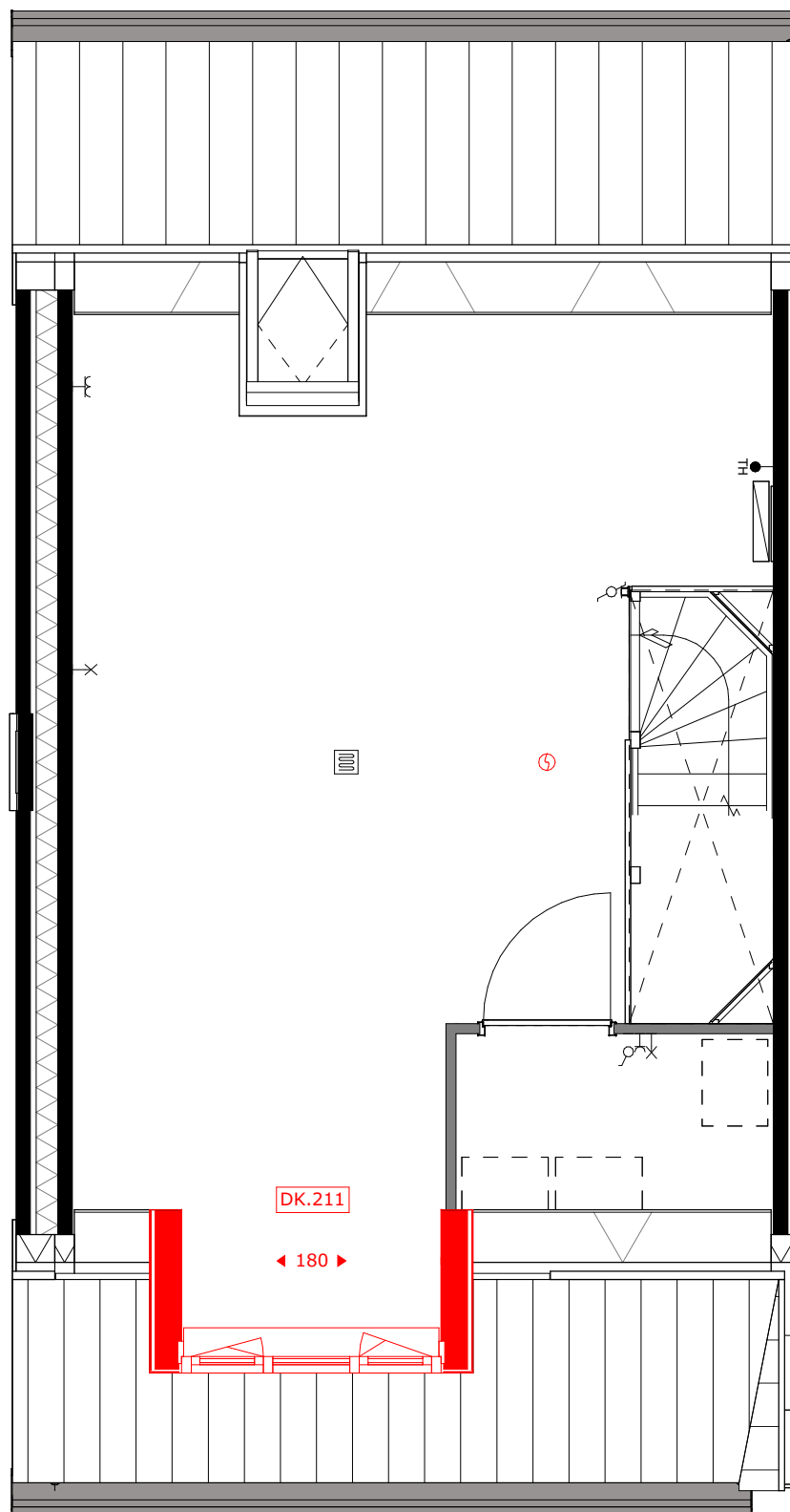
DK.211 = dakkapel voorgevel (breedte c.a. 1.8m)
