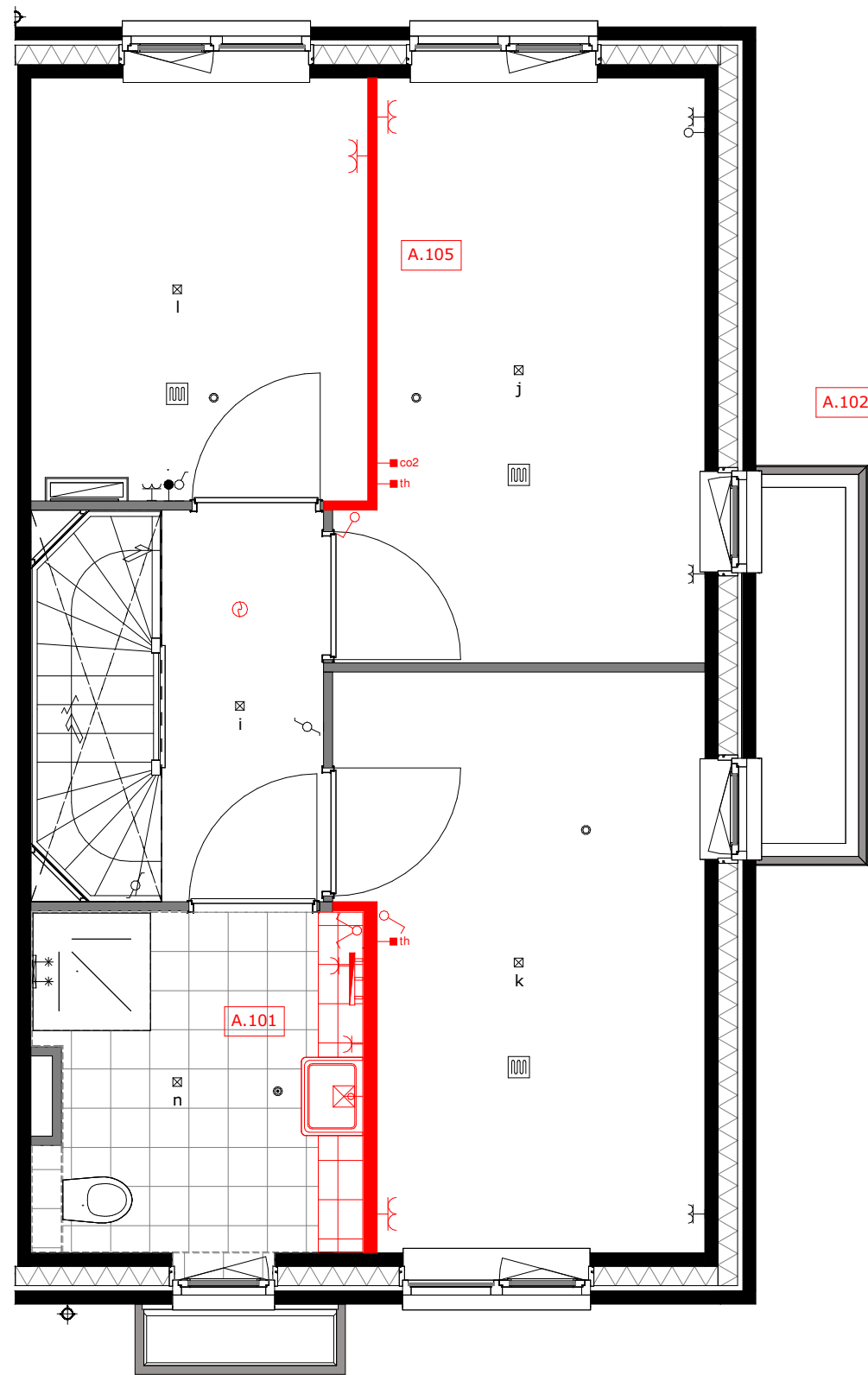
A.101 = vergroten badkamer ca. 35cm A.106 = verplaatsen wand slaapkamer 1 en 3
