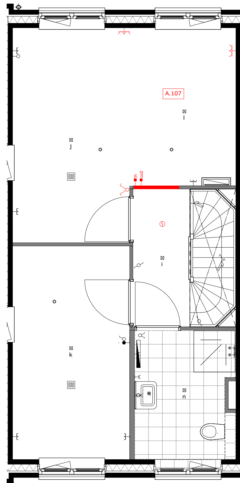
A.107 = slaapkamer 1 en 3 samenvoegen
