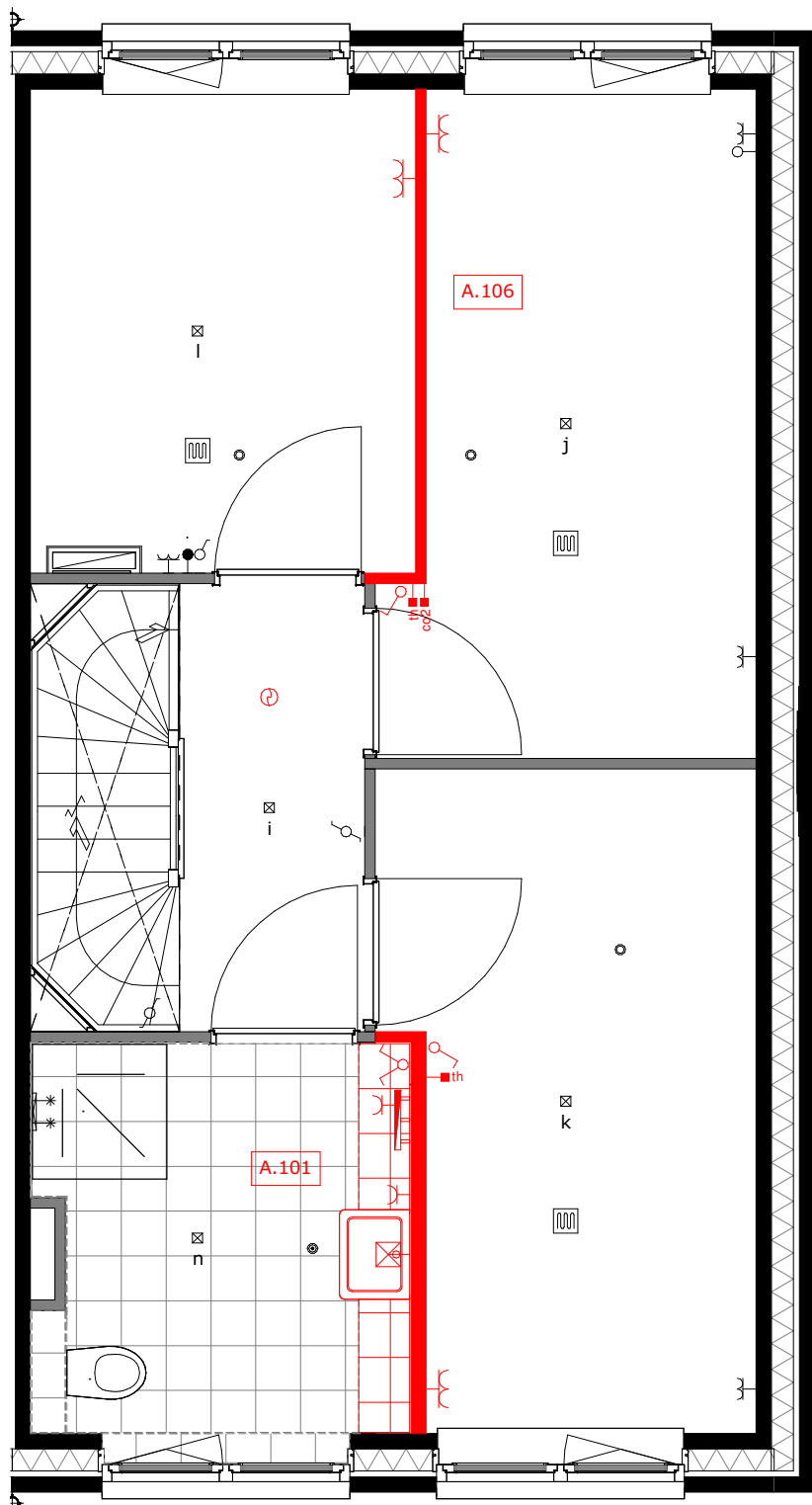
A.101 = vergroten badkamer ca. 35cm A.106 = verplaatsen wand slaapkamer 1 en 3
