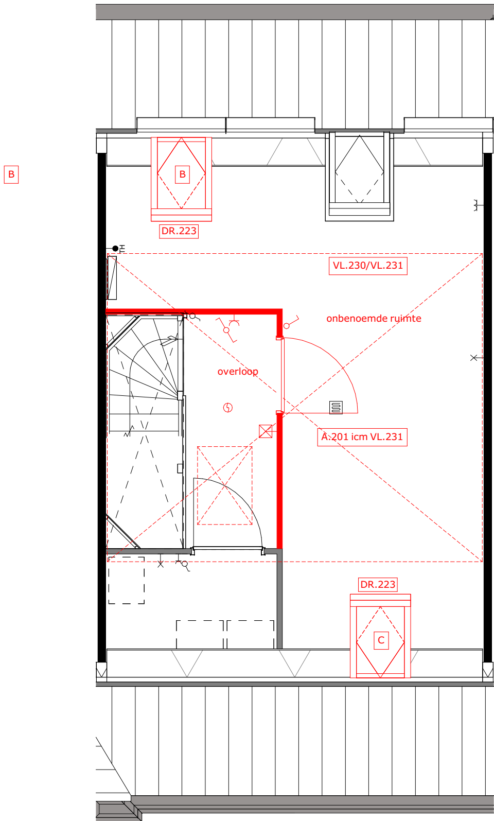
A.201 = zolderindeling (alleen in combinatie met VL.231) DR.223 = houten tuimeldakraam VL.230 = vliering (onafgewerkt) VL.231 = vliering afgewerkt
